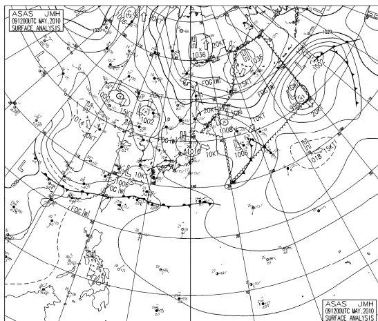
地上天気図 9日21時
