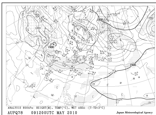
850hpa面高度・気温・湿数 9日21時
