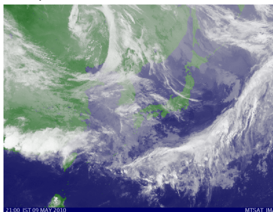
赤外線雲画像 9日21時
